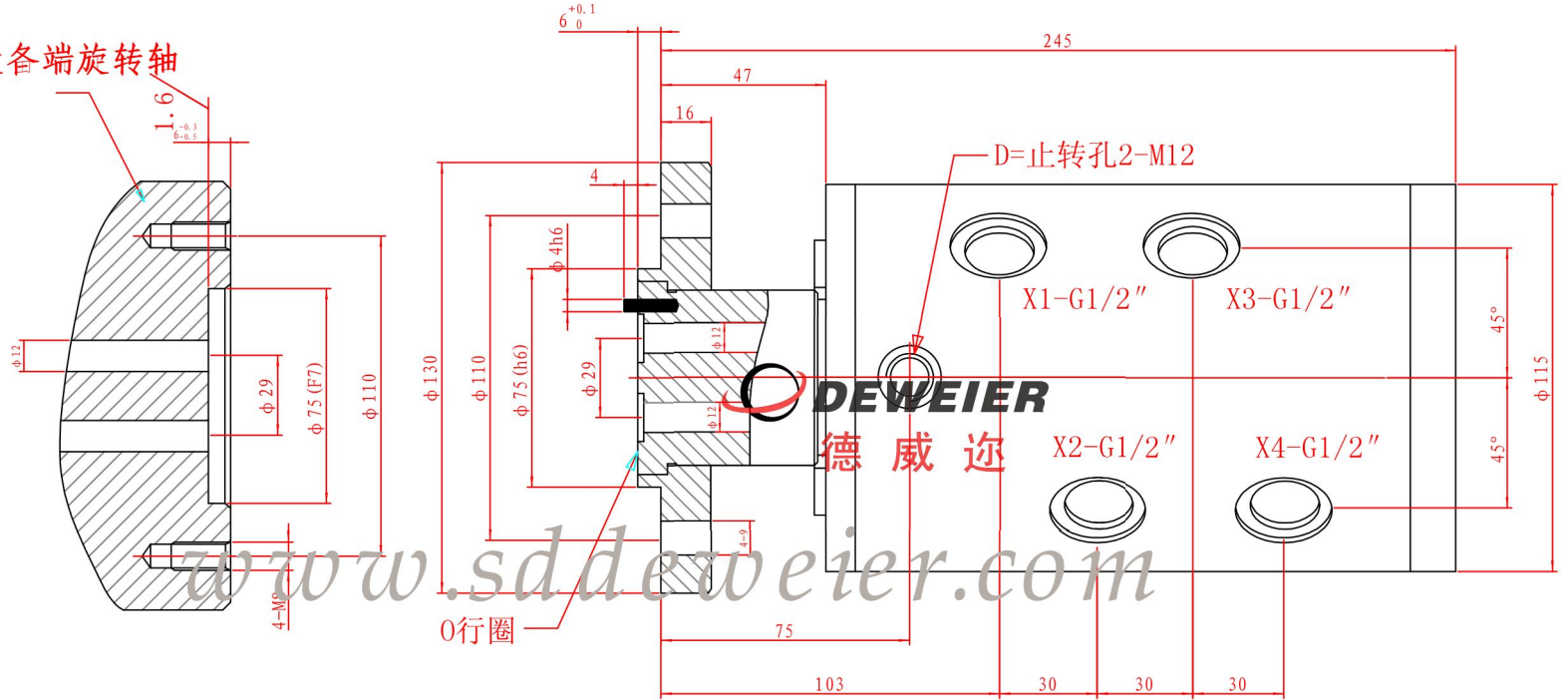
液压四通道旋转接头-DRF04015
